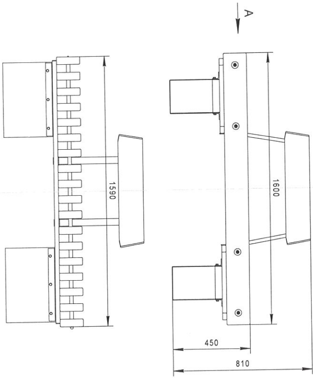
Рисунок 2 - Габаритные размеры изделия
